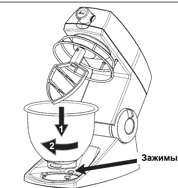
Рис.5 Дежу ставят в миксер и поворачивают, чтобы зафиксировать зажимами.
