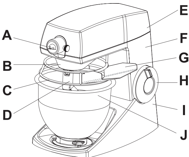
Рис. 1 Конструкция миксера
